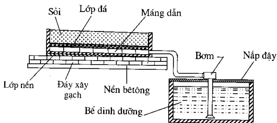
Hình 2.11. Hệ thống trồng cây trong sới sử dụng hệ thống tưới ngầm (cung cấp trực tiếp)
