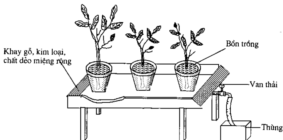
Hình 3.6. Tưới ngầm trong khay rộng
