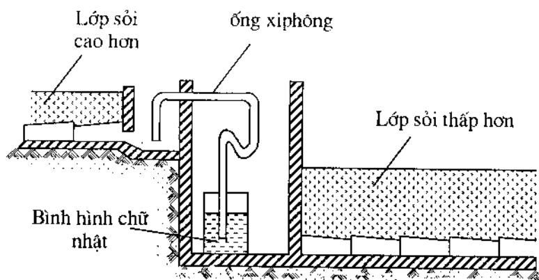
b) Phương pháp lựa chọn chỗ nối bằng ống xìphông tự động
